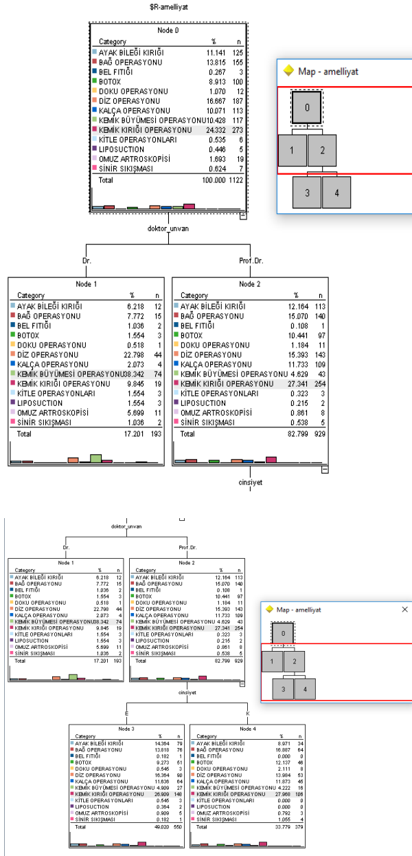
Şekil 2. Chaid Karar Ağacı Algoritması
